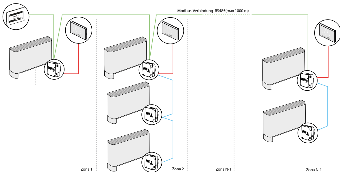
Systemlösung mit FCL-Boxen und GLF-Gittern
