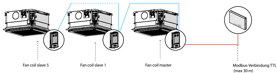
Systemlösung mit FCL-Boxen und GLF-Gittern
